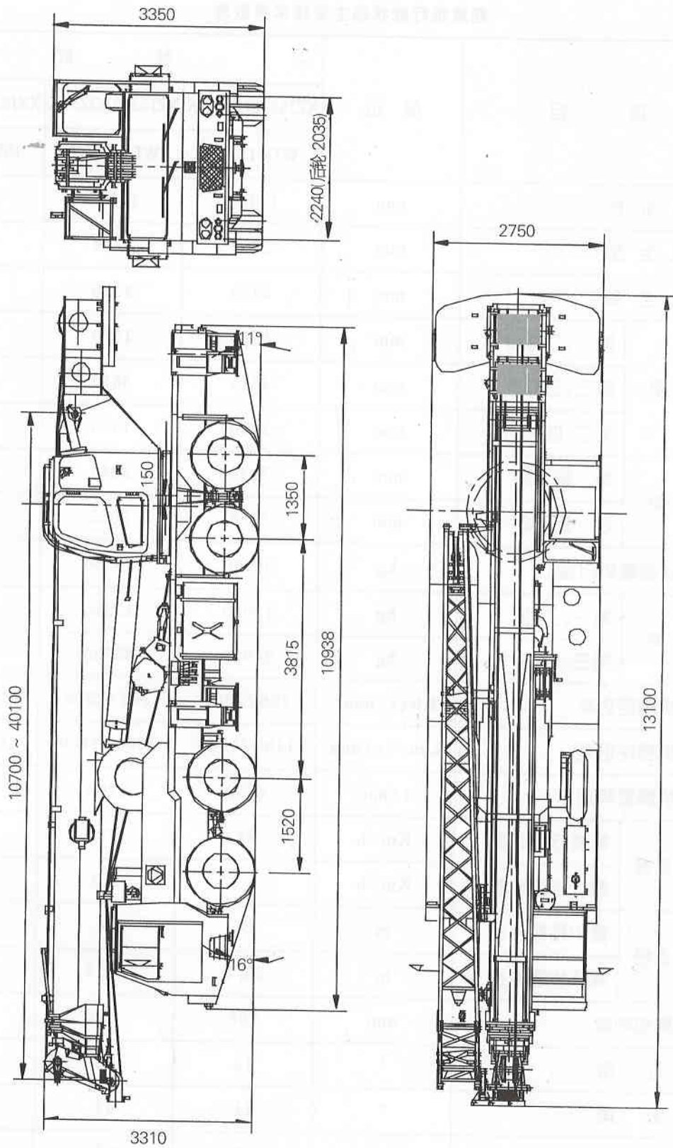
图 3-1 整机外形图
